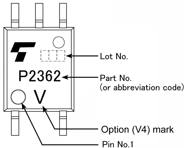
Fig. 16.4 Marking Example(Note)
