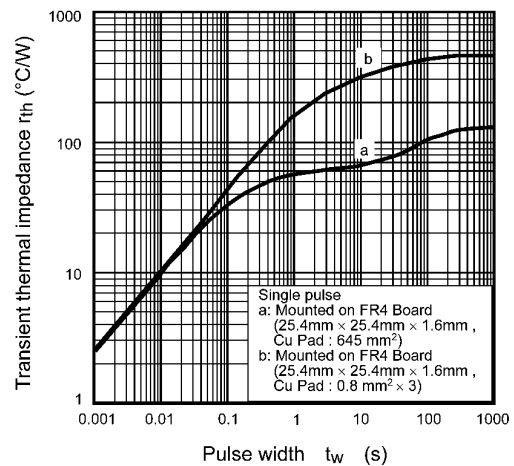
Fig. 7.12 r_{th} - t_w
