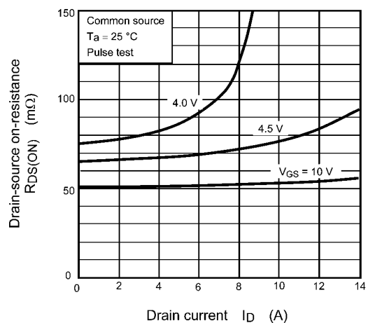
Fig. 7.4 R_{DS(ON)} - I_D
