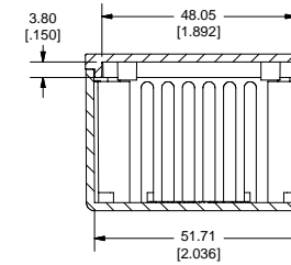
SECTION D-D
