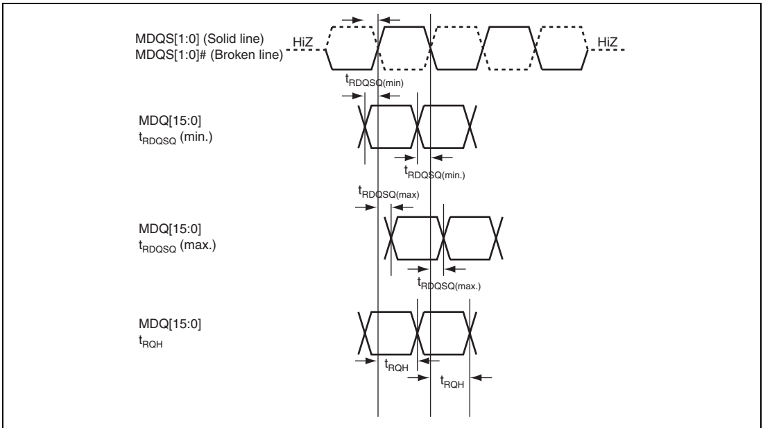
Figure 52.29 DQ Input Waveform Limitation on DQS (Read)
