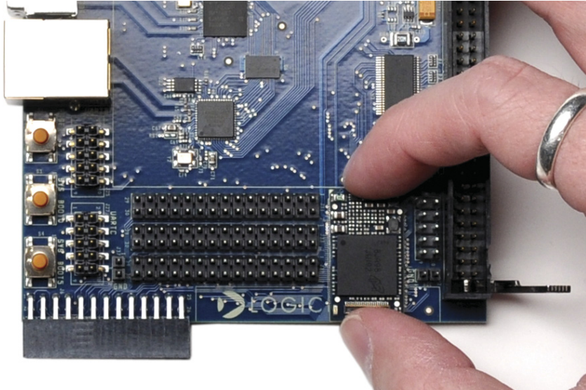
Figure 2.2 – Align the SOM over the Baseboard
