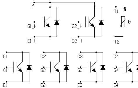
Schaltbild
